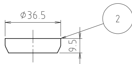
寸法 30
