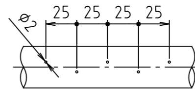
洗体用放水管穴明け詳細図
