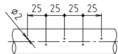
洗体用放水管穴明け詳細図
