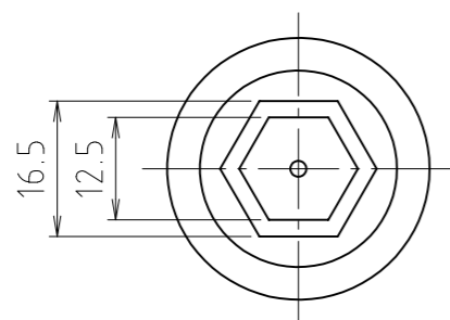
寸法 20
