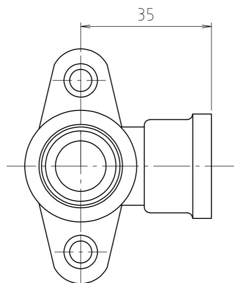
寸法 13
