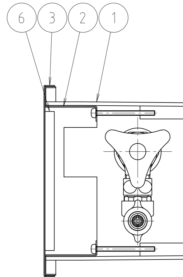
断面図
